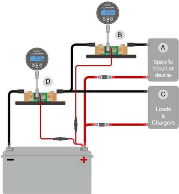
Ejemplo de conexión de un sistema con un monitor de baterías principal, junto con otro monitor de baterías que se ha configurado como contador CC y monitoriza un dispositivo o circuito específico. Un monitor de baterías se usa como contador CC (B) y el otro como monitor de baterías (D).
