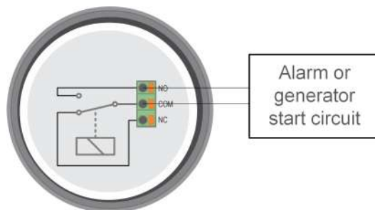
Diagrama de cableado interno del monitor de baterías con el relé en estado desactivado conectado a un circuito externo de alarma o arranque de un generador.
